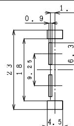
基板孔参考寸法
