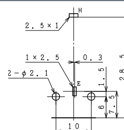
基板孔参考寸法
