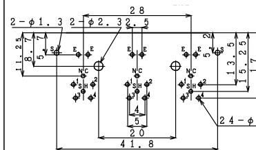
基板孔参考寸法
